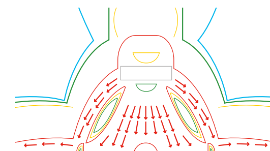
FLUX D'AIR DU CYCLONE 360
